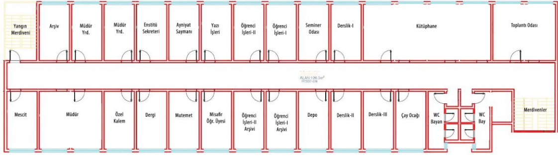
Resim 16: Enstitü Mimari Planı
