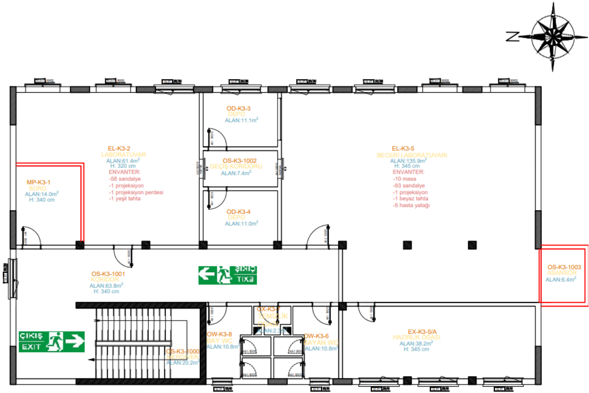
HEMŞİRELİK FAKÜLTESİ 2. KAT PLANI ÖLÇEK 1/50
