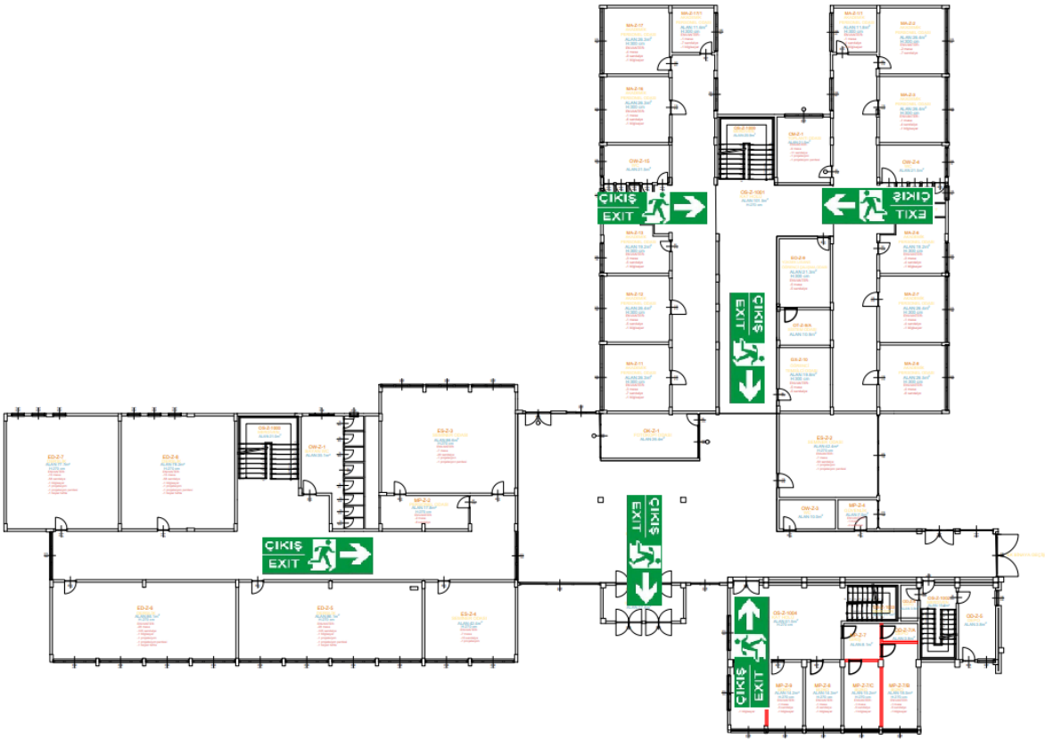
HEMŞİRELİK FAK ZEMİN KAT PLANI
