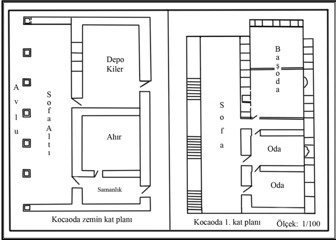
Şekil 4.1. Kocaoda'nın (Bakibey Konağı) Planı.
