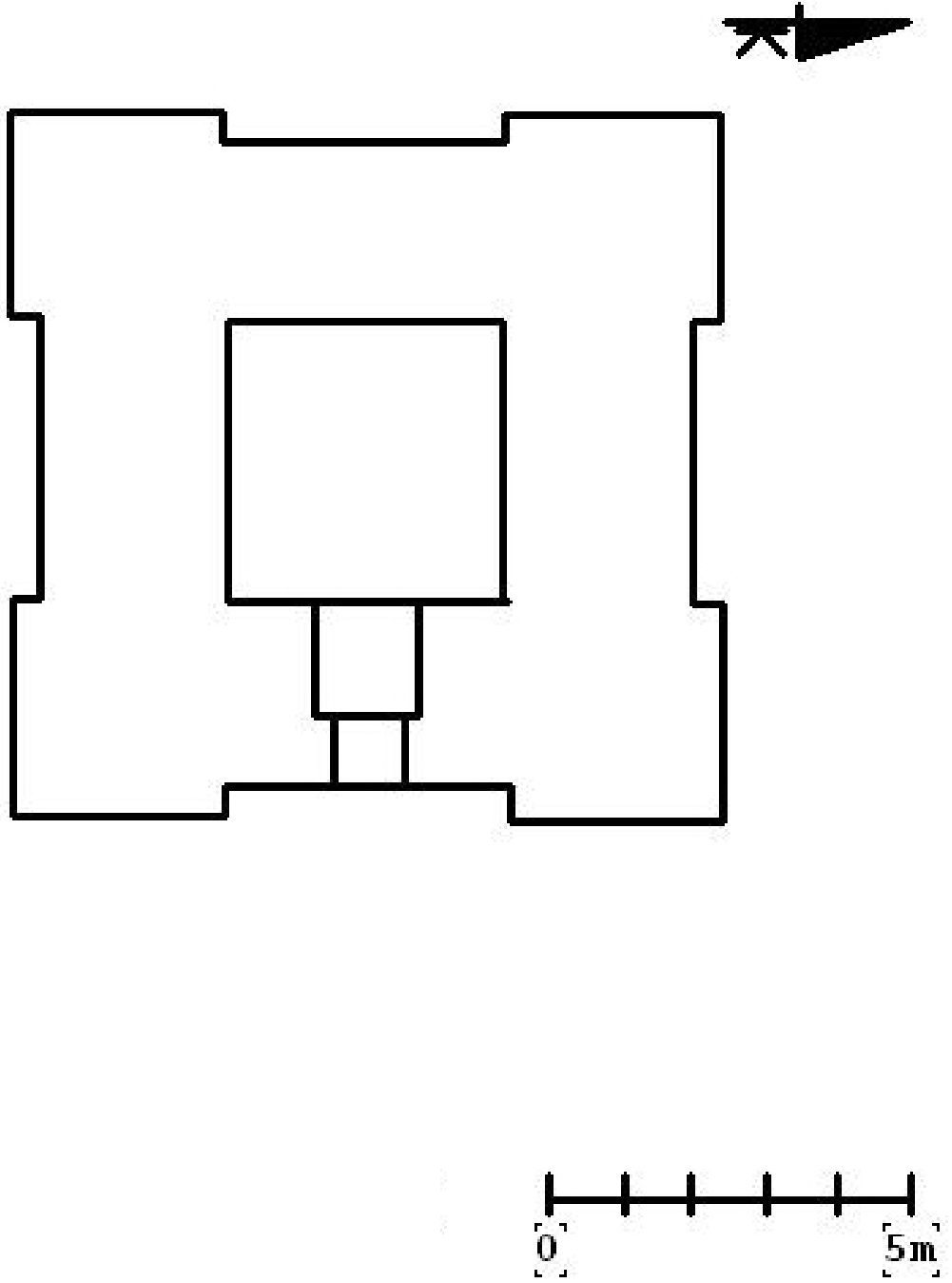
Çizim 11: Çavuştepe Aşağı Kale Tapınak Planı
