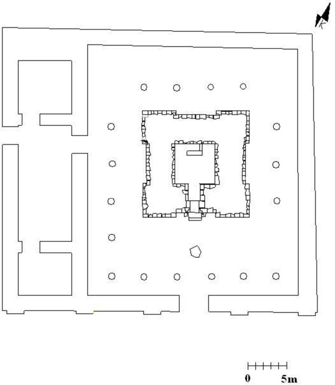
Çizim 20: Altıntepe Tapınak Planı
