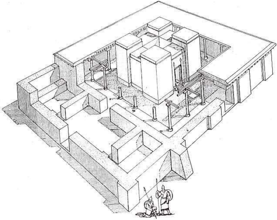
Çizim 23: T. Özgüç Tarafından Yapılan Altintepe Tapınağı Yeniden Kurma Denemesi
