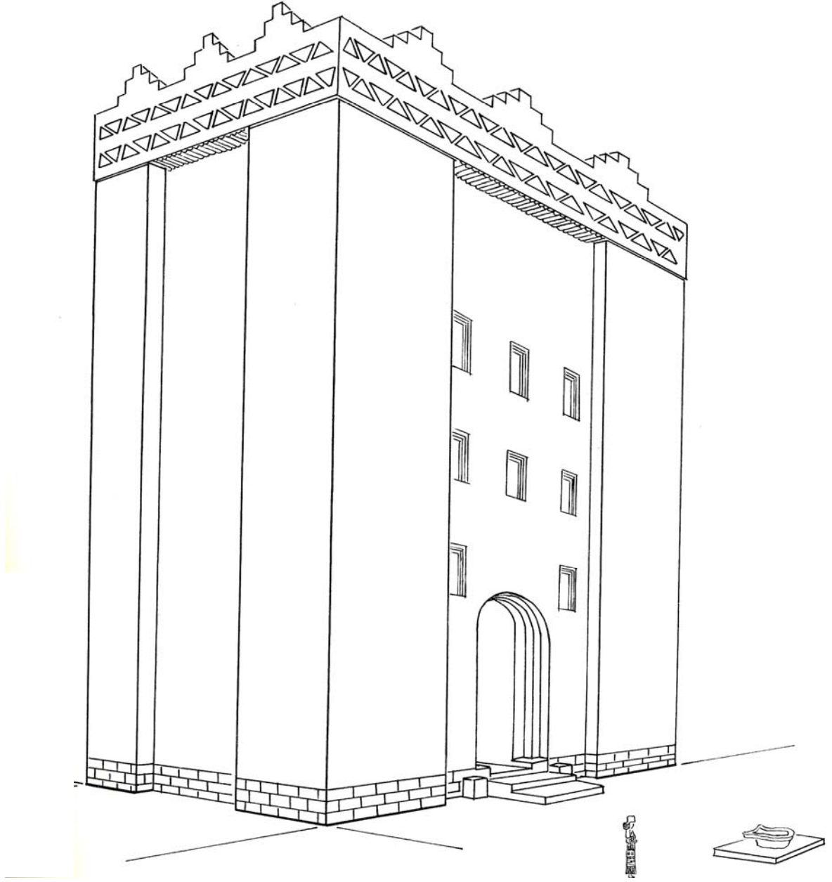
Çizim 24: E.Akurgal Tarafından Yapılan Urartu Tapınağı Yeniden Kurma Denemesi
